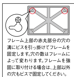
枠の吊下げ穴の位置で壁にビスを打ち枠を固定します。
